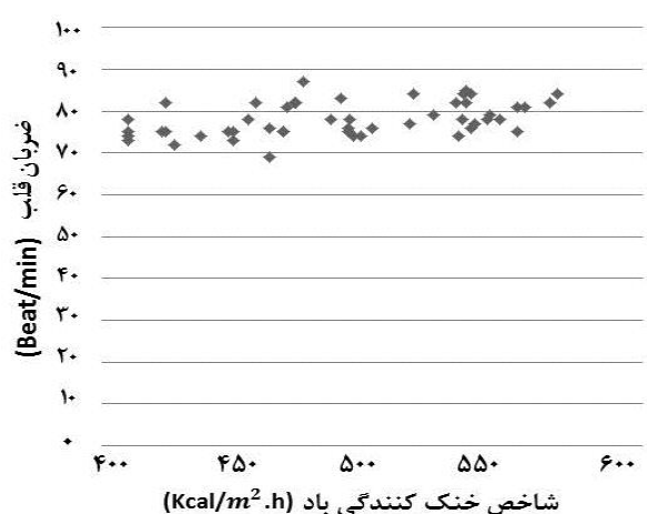
شکل ۳: نمودار پراکنش ارتباط بین شاخص خنک‌کنندگی باد با پاسخ‌های فیزیولوژیکی
