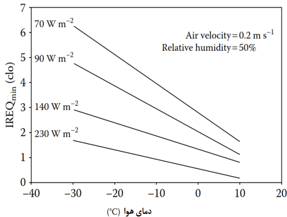
شکل ۲: نمودارهای تعیین حداقل عایق مورد نیاز (IREQ min) و عایق مورد نیاز برای حفظ تعادل حرارتی بدن (IREQ neutral)
