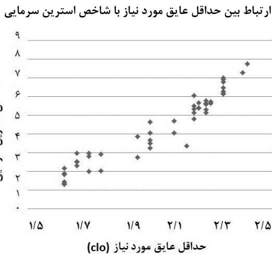
شکل ۵: نمودار پراکنش ارتباط بین حداقل عایق مورد نیاز با پاسخ‌های فیزیولوژیکی
