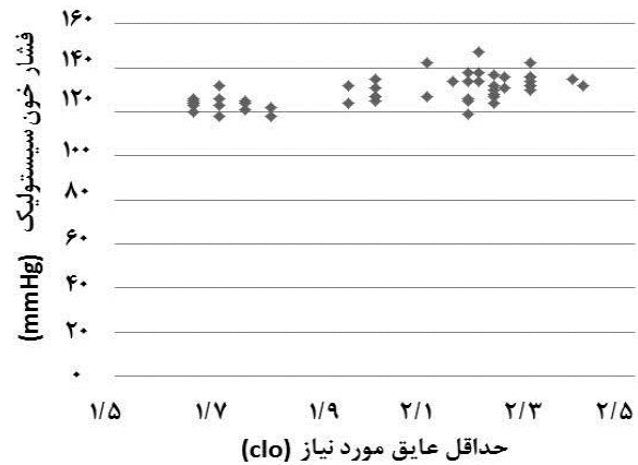
ارتباط بین حداقل عایق مورد نیاز با فشار خون سیستولیک
