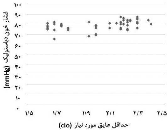
ارتباط بین حداقل عایق مورد نیاز با فشار خون دیاستولیک
