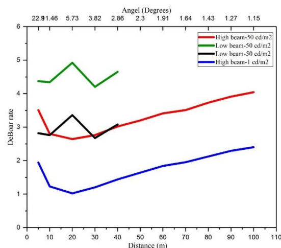
شکل ۶: میانگین خیرگی آژاردهنده چراغ خودروها در زوایا و فواصل مختلف اندازه‌گیری در حالت نورپایین و نوربالا
