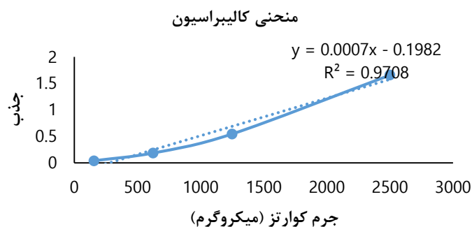
شکل ۱: منحنی کالیبراسیون کوارتز
