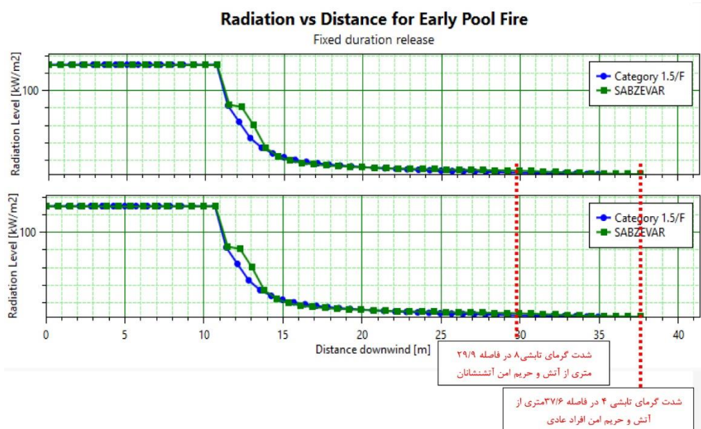
شکل ۵. نمودار شدت تابش بر حسب فاصله برای آتش استخری اولیه برای مخزن ۱۲۰۰۰ m 3 و ۲۳۶۰۰ m 3
