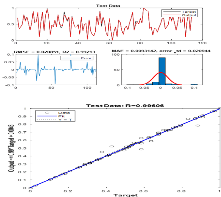
شکل ۴: نمودارهای داده‌های آزمایشی به روش خوشه‌بندی کاهشی و معیارهای ارزیابی عملکرد
