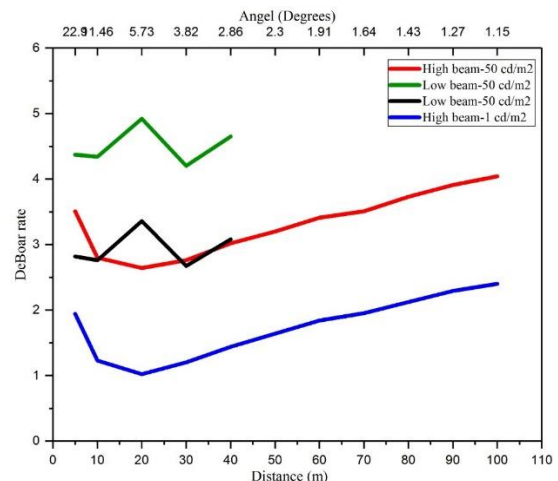
شكل ۶: ميانگين خيريگي آزاردهنده چراغ خودروها در زوايا و فواصل مختلف اندازه‌گيري در حالت نورپايين و نوربالا
