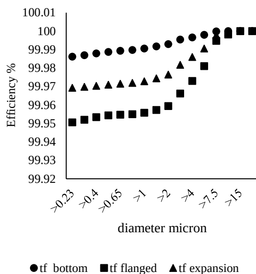
شکل ۷: راندمان در قطرهای مختلف ذرات بعد از گذشت چند دوره فیلتراسیون دیگر
