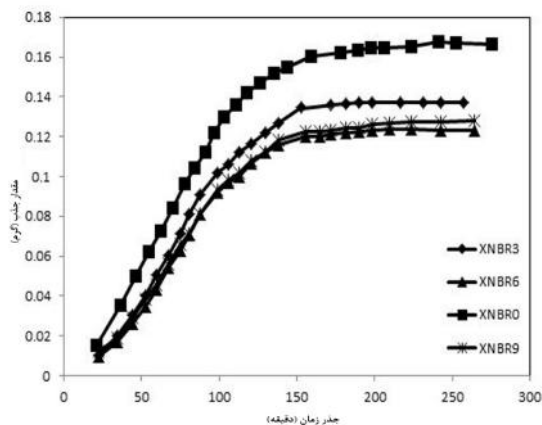
شکل ۱- منحنی تورم نانو کامپوزیت-تراکلریدکربن بر
