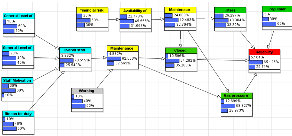
شکل ۱. حل مدل پیشنهادی توسط نرم‌افزار آجینا ریسک
