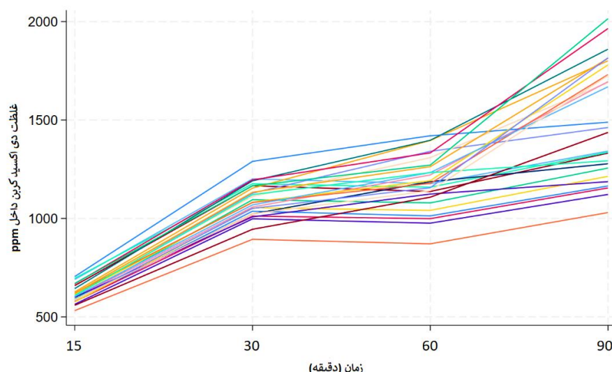
شکل ۱: روند تغییرات غلظت \text{CO}_2 در طول زمان تدریس
