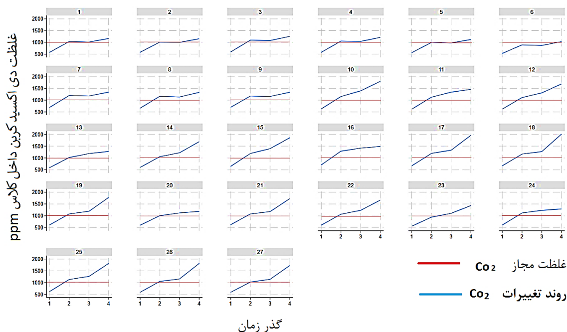
شکل ۲: مقایسه روند تغییرات غلظت \text{CO}_2 با حد استاندارد WHO (۱۰۰۰ قسمت در میلیون) در طول زمان تدریس به تفکیک کلاس‌ها
