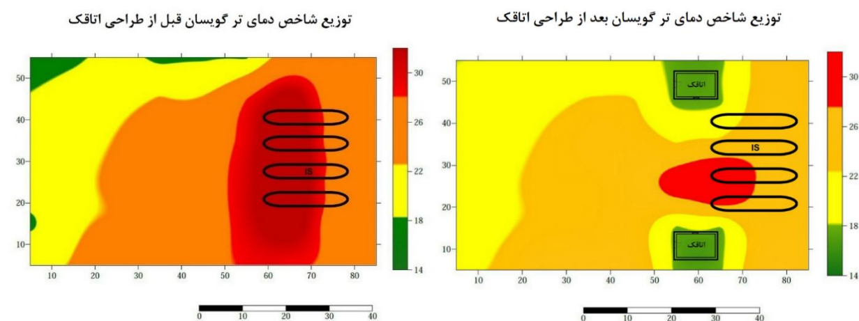
شکل ۳. نقشه ی توزیع شاخص دمای تر گوی سان (WBGT) قبل و بعد از طراحی اتاقک
