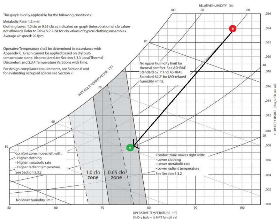
شکل ۲. تحول سایکرومتریک سرمایش و رطوبت گیری جهت تأمین آسایش حرارتی کارکنان در اتاقکها مطابق با استاندارد ASHRAE 55
