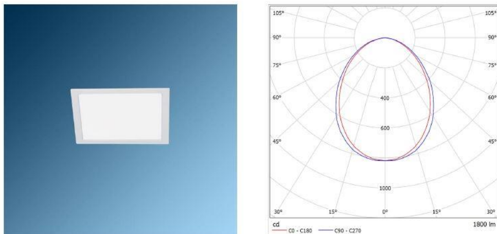
شکل ۶. شکل شماتیک نحوه‌ی قرارگیری چراغ‌های LED داخل اتاقک و محدوده‌ی رنگ‌بندی شدت روشنایی داخل اتاقک
