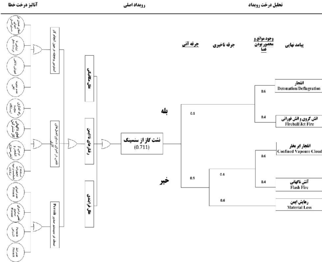
شکل ۱- خروجی آنالیز نشتی گاز از سنسورینگ در ایستگاه‌های TBS با استفاده از روش آنالیز پایبونی
