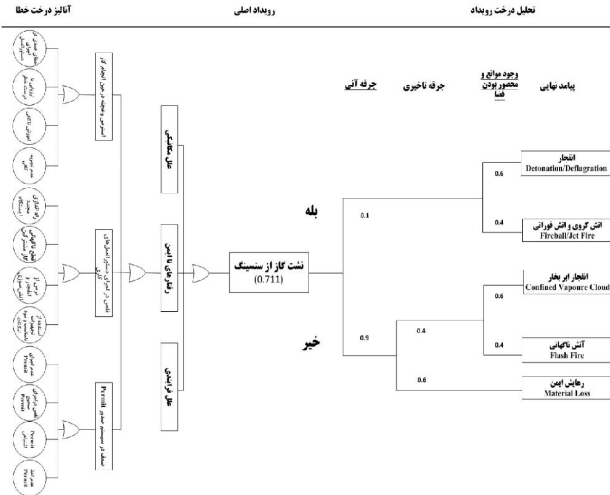
شکل ۱- خروجی آنالیز نشتی گاز از سنسینگ در ایستگاه‌های TBS با استفاده از روش آنالیز پایونی
