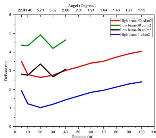
شکل ۶: میانگین خیرگی آژاردهنده چراغ خودروها در زوایا و فواصل مختلف اندازه‌گیری در حالت نورپایین و نوربالا
