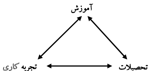
شکل ۱- مثلث OSH
