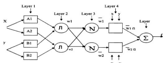
نمودار ۲: نمونه ساختار ANFIS
