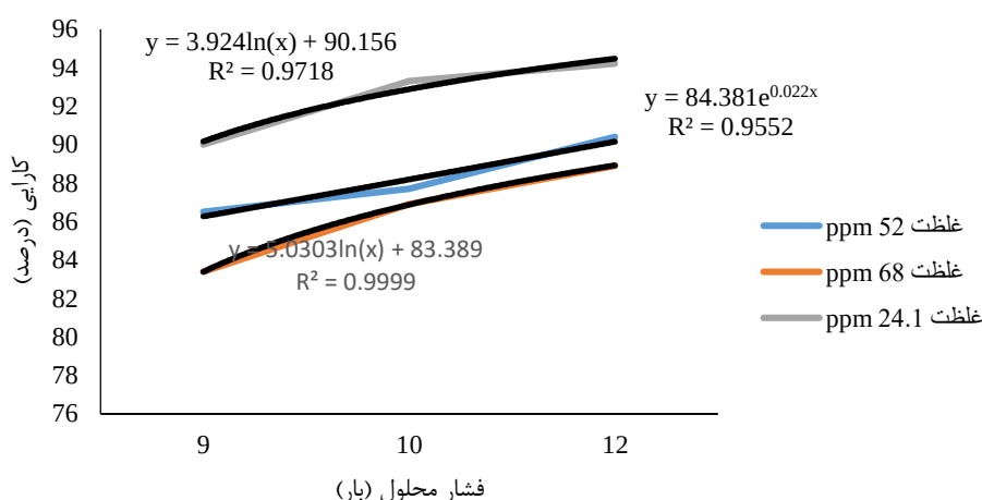
نمودار ۲: کارایی حذف گاز آمونیاک نسبت به فشار محلول مایع شست‌وشودهنده با دو نازل ۲۰ میکرونی و مایع شست‌وشودهنده آب و اسید سولفوریک
