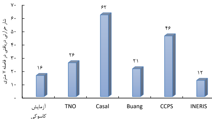
نمودار ۱: مقایسه شار حرارتی دریافتی به وسیله هدف در فاصله ۷ متر از مخزن با استفاده از مدل‌های تجربی
