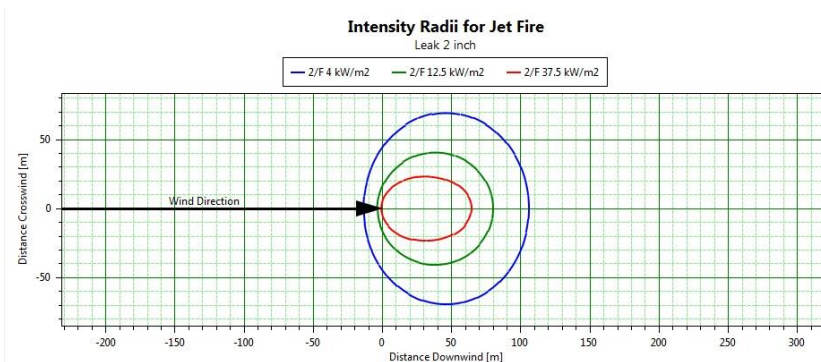
شکل ۱: نتایج سناریوی آتش فورانی
