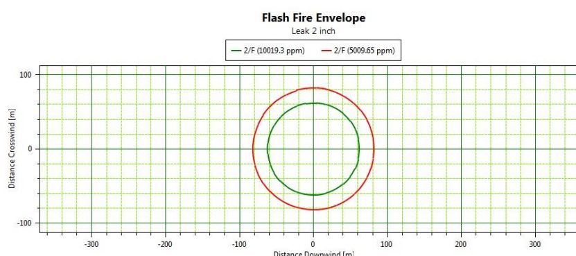
شکل ۳: نتایج سناریوی آتش ناگهانی
