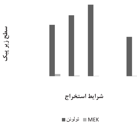
تصویر ۳: سطح زیر پیک دو ماده در شرایط مختلف استخراج (۱): ۶۰ دقیقه، ۵۰ درجه سانتی‌گراد، بانمک ۲: ۳۰ دقیقه، ۵۰ درجه سانتی‌گراد، بانمک ۴: ۳۰ دقیقه، ۳۰ درجه سانتی‌گراد، بانمک ۵: ۳۰ دقیقه، ۳۰ درجه سانتی‌گراد، بدون نمک ۶: ۳۰ دقیقه، ۳۰ درجه سانتی‌گراد، بدون نمک ۷: ۶۰ دقیقه، ۳۰ درجه سانتی‌گراد، بدون نمک ۸: ۶۰ دقیقه، ۵۰ درجه سانتی‌گراد، بدون نمک
