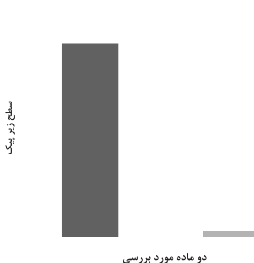
تصویر ۴: سطح زیر پیک دو ماده در دما و زمان بهینه استخراج
