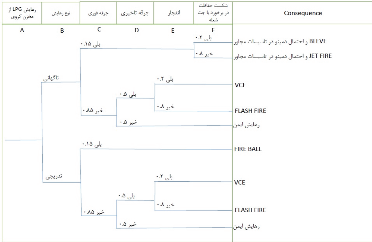
تصویر ۳: درخت رویداد ترسیم‌شده مربوط به رهائش گاز LPG از مخزن کروی در روش Bowti
