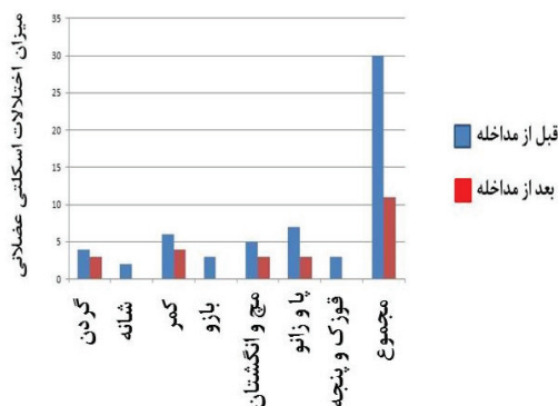
تصویر ۱: مقایسه تعداد موارد اختلالات اسکلتی عضلانی قبل و بعد از مداخله
