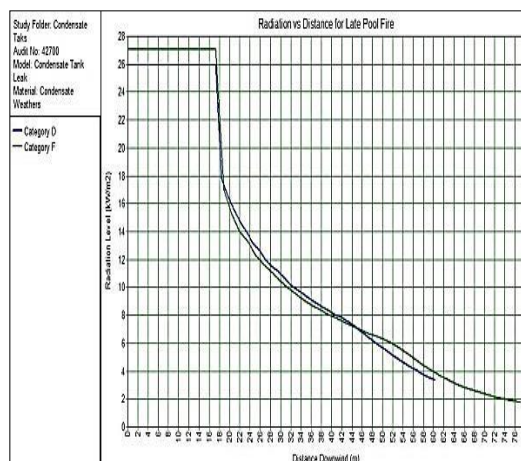
شکل ۳: مقدار تشعشعات بر حسب فاصله در نشستی مخزن
